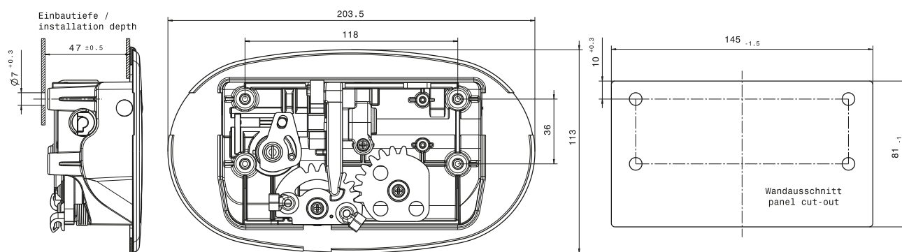
Abb. / Illus. 11 mit geschlossenem Griff / with closed handle
