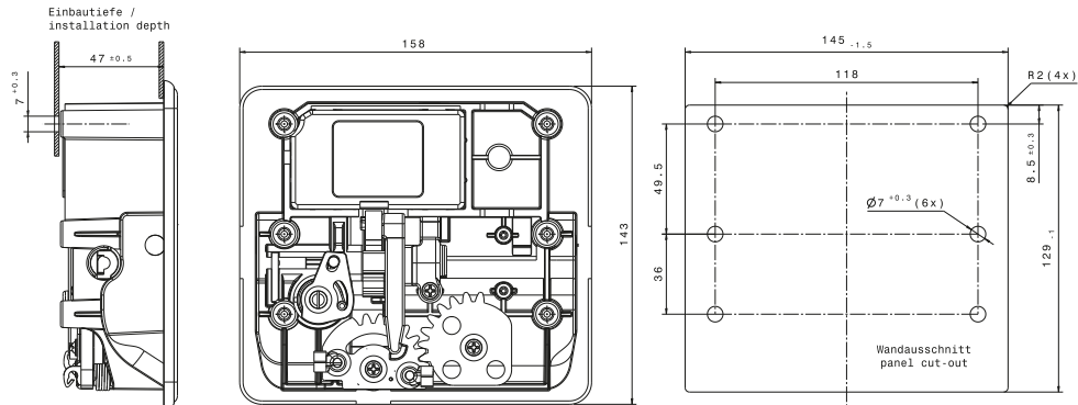
Abb. / Illus. 3 mit geschlossenem Griff / with closed handle
