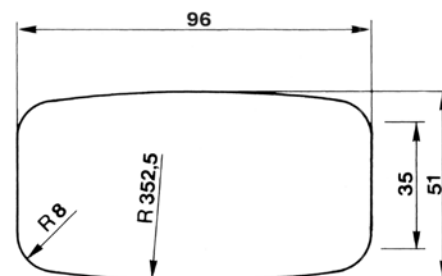
Einbauöffnung/assembly aperture
